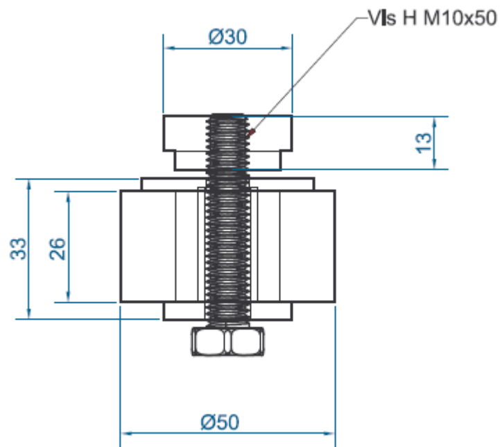
Olive nylon sur cage à rouleaux
